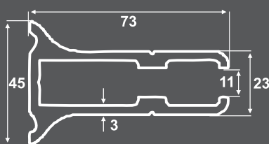
SD-6011 | 11,50kg ΠΡΟΦΙΛ ΔΑΠΕΔΟΥ ΤΖΑΜΙΟΥ 73x45mm On floor profile for glass 73x45mm
