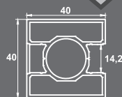
SD-7005N ΚΟΛΩΝΑ ΤΕΤΡΑΓΩΝΗ 40x40 Squared Column 40x40
